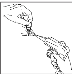
Limpar o filtro assoprando com ar sob pressão
