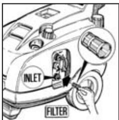
Extraer el filtro del empaque del ingreso de agua
